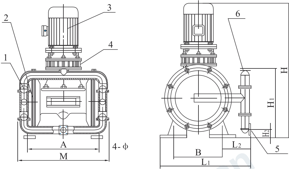
立式安装尺寸与外形尺寸
