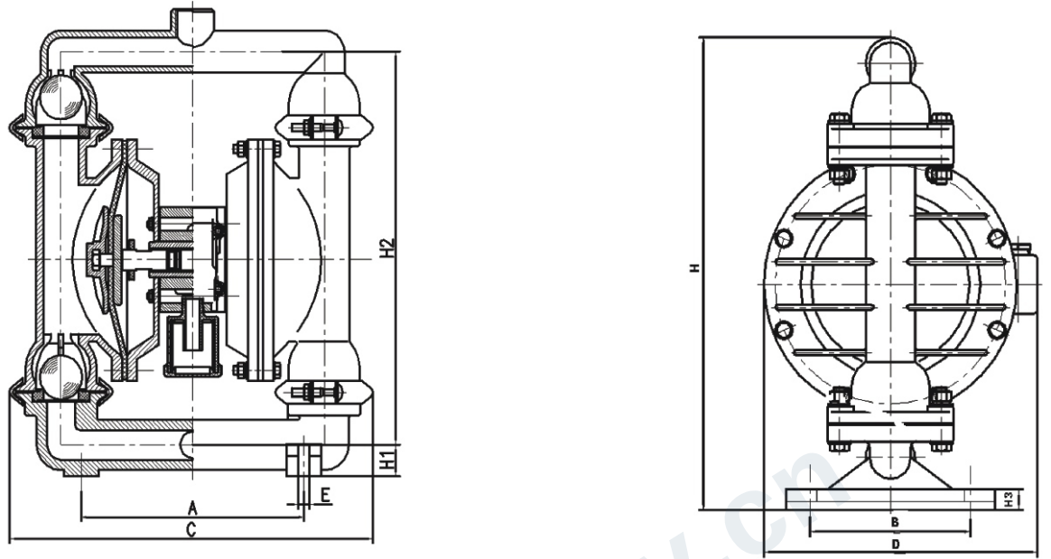
主要外形尺寸表 Tables of setting data
